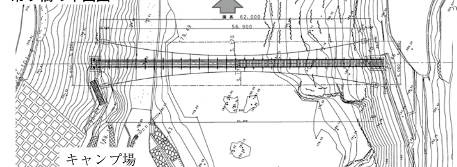
吊り橋の平面図
