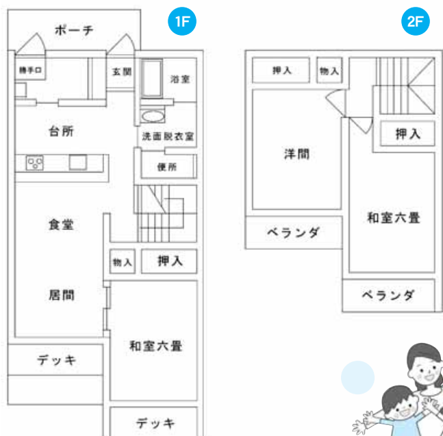
喰田町営住宅の平面図
